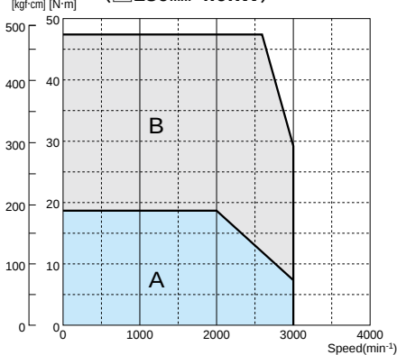
TS4927 N□□□□ E215 (□220mm 11.0kW)
