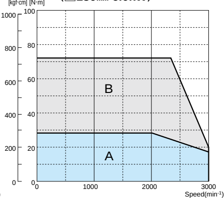
TS4920 N□□□□ E215 (□220mm 15.0kW)
