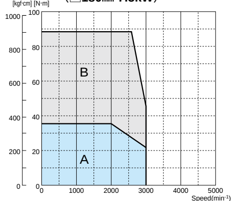
TS4889 N□□□□ E225 (□180mm 7.5kW)
