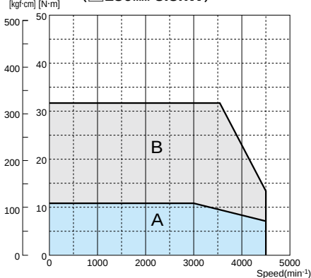
TS4884 N□□□□ E225 (□180mm 4.0kW)
